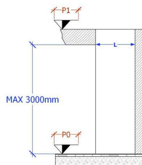
PROSPETTO
