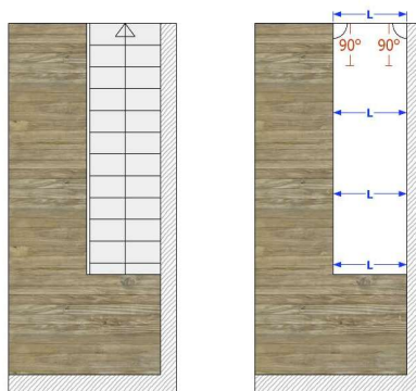
PIANTA
